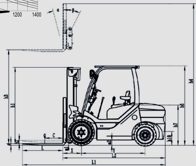
KION standard chassis
